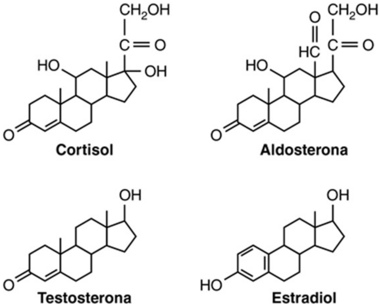
FIGURA 75-3 Estructura química de diversas hormonas esteroideas.
