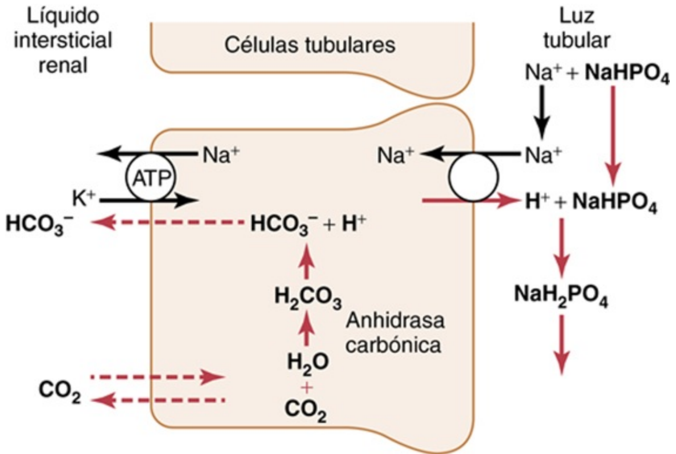
FIGURA 31-7 Amortiguación de iones hidrógeno secretados por el fosfato filtrado ( \text{NaH}_2\text{PO}_4^- ). Obsérvese que se devuelve un nuevo ion \text{HCO}_3^- a la sangre por cada \text{NaH}_2\text{PO}_4^- , que reacciona con un \text{H}^+ secretado.
