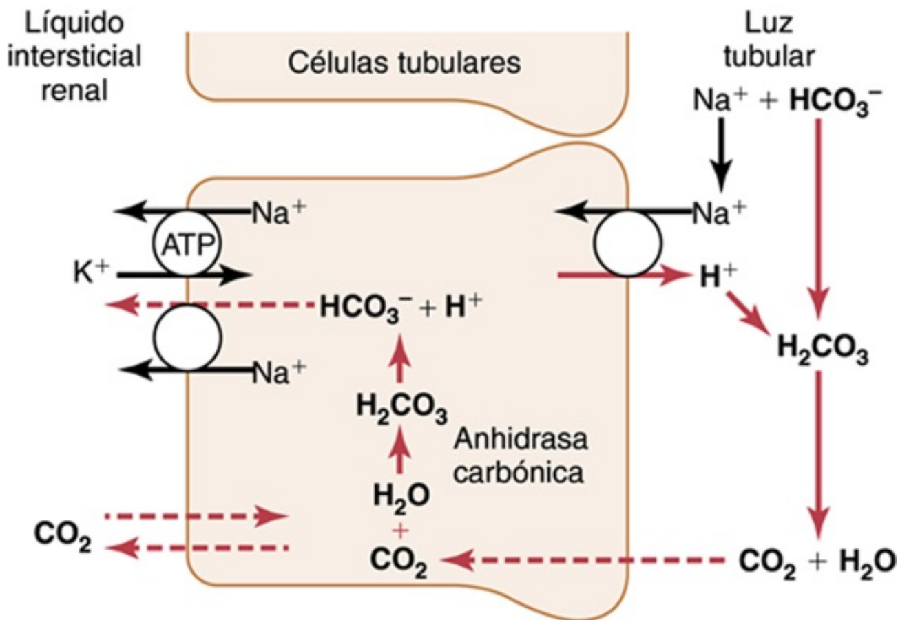
FIGURA 31-5 Mecanismos celulares de: 1) secreción activa de H^+ en el túbulo renal; 2) reabsorción tubular de iones HCO_3^- mediante la combinación de H^+ para formar ácido carbónico, que se disocia para formar dióxido de carbono y agua, y 3) reabsorción de ion sodio en intercambio por H^+ secretados. Este patrón de secreción de H^+ tiene lugar en el túbulo proximal, el segmento ascendente grueso del asa de Henle y la primera parte del túbulo distal.
