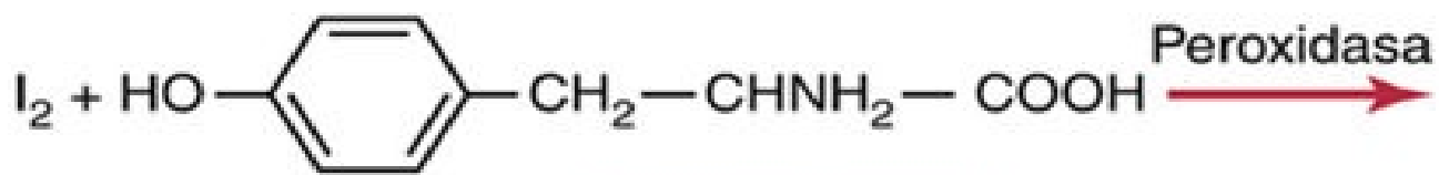
Tirosina
